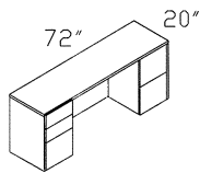
RU-7220CR Kneespace Credenza
