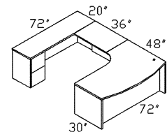
RU-EUBTCC L/R 'U' W/Bow Top W/Computer Corner-Left or Right
