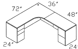
RU-ELCC L/R 'L' W/Corner Credenza -Left or Right
